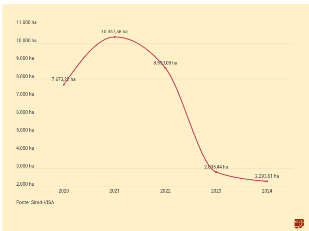
Gráfico 1 - Desmatamento (ha) por ano nas áreas monitoradas (2020-2024)
