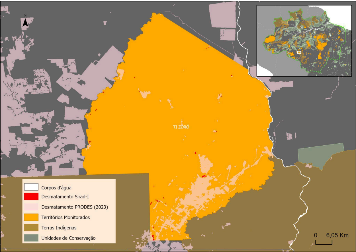
Mapa 2 - Desmatamento na Terra Indígena Zoró (2023 - 2024)
