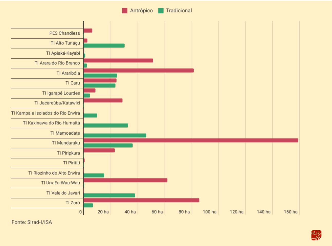
Gráfico 2 - Desmatamento (ha) por distinção de uso nas áreas monitoradas (2024)
