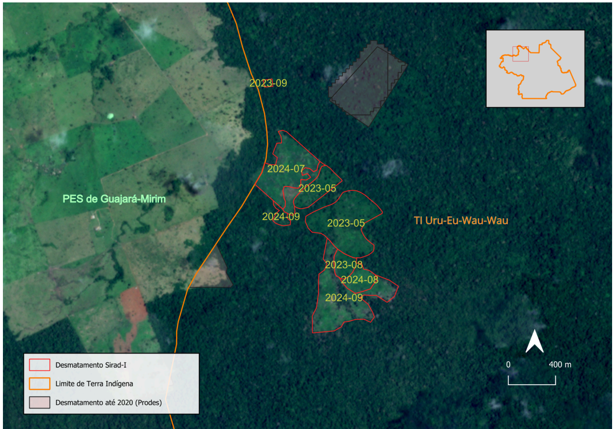
Mapa 11 - Desmatamento na borda com o Parque Estadual Guajará-Mirim
