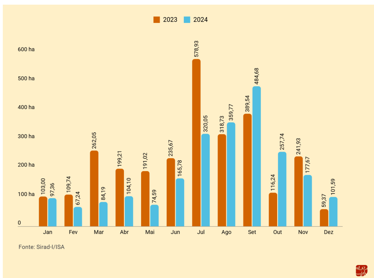
Gráfico 3 - Desmatamento (ha) por mês nas áreas monitoradas (2023 e 2024)
