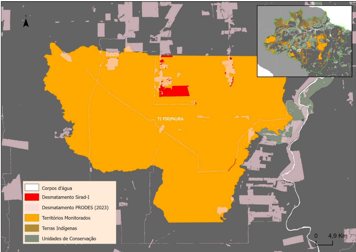
Mapa 7 - Desmatamento na Terra Indígena Piripkura (2023 - 2024)
