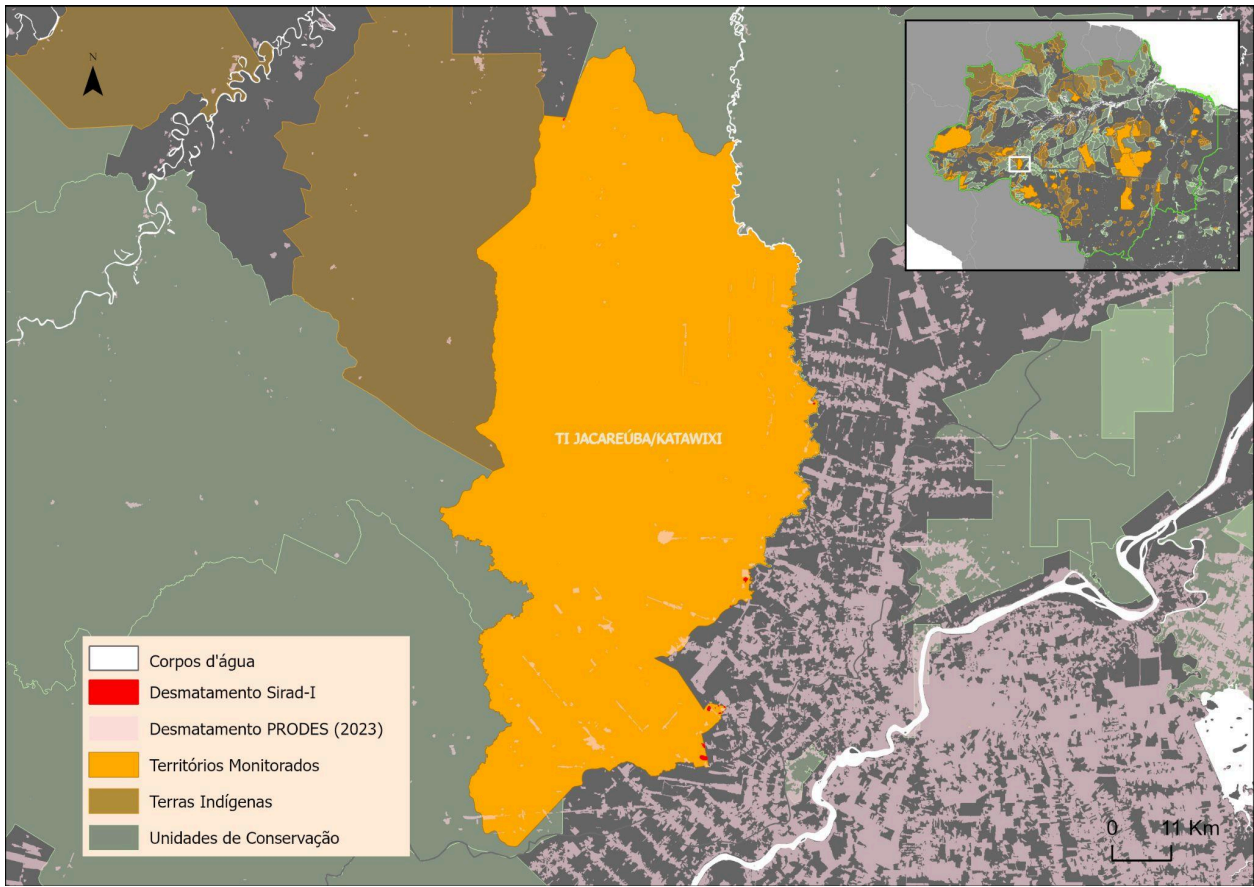
Mapa 9 - Desmatamento na Terra Indígena Jacareúba-Katawixi (2023 - 2024)
