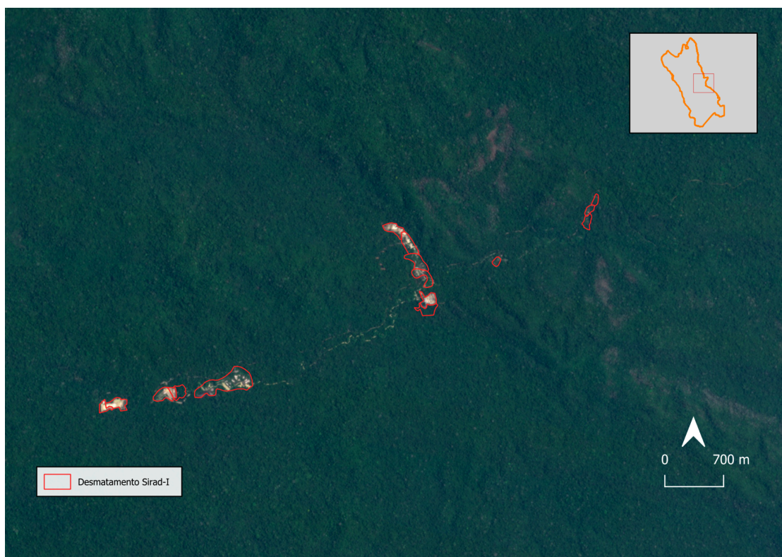
Mapa 6 - Garimpo próximo ao Igarapé Marupazinho (Setembro, 2024)
