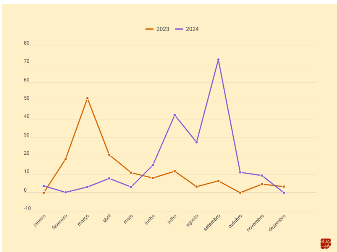
Gráfico 4 - Evolução das áreas de garimpo na Terra Indígena Mundurucu (2023 e 2024)
