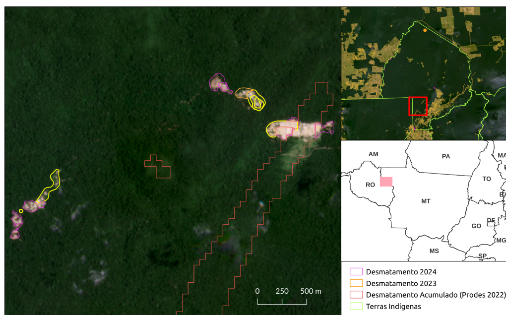
Mapa 3 - Desmatamentos relacionados à atividades de mineração ilegal na TI Zoró (2024) 14
