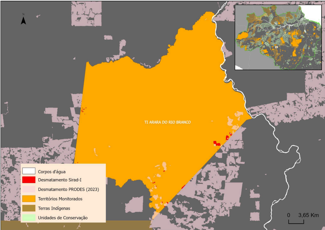
Mapa 12 - Desmatamento na Terra Indígena Arara do Rio Branco (2023 - 2024)
