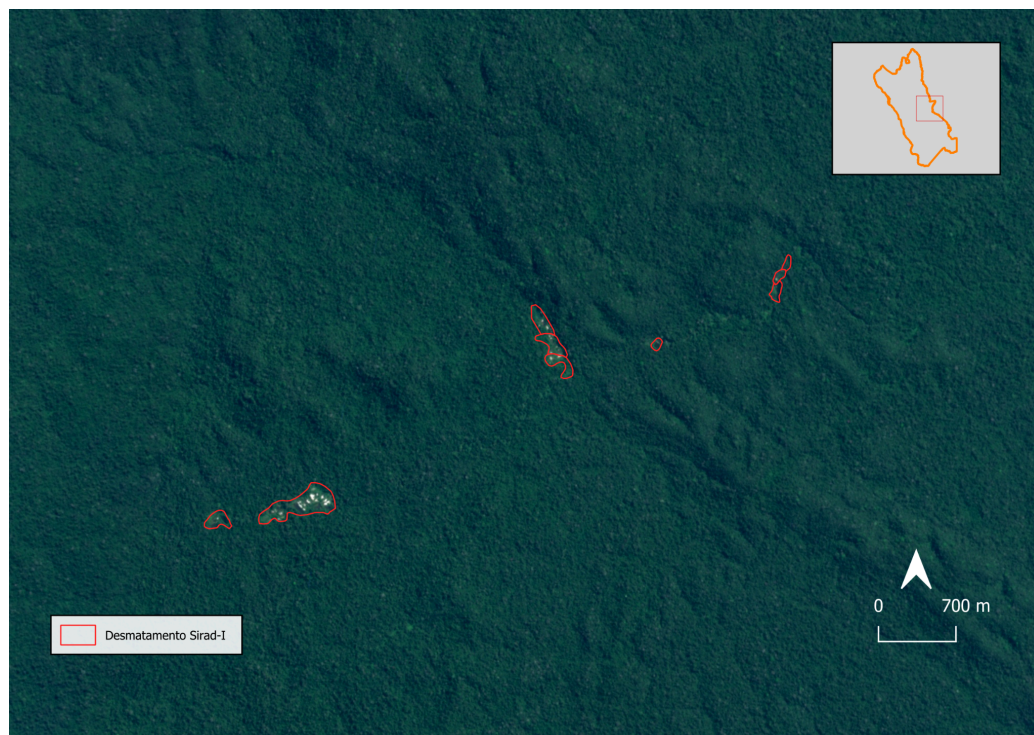
Mapa 5 - Garimpo próximo ao Igarapé Marupazinho (Maio, 2024)
